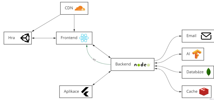
Obrázek 3.1: Architektura aplikace.
